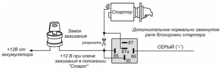
Схема подключения СЕРЫГО провода для блокировки цепи зажигания автомобиля:
