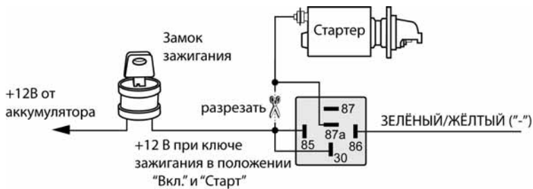
Схема подключения ЗЕЛЕНОГО/ЖЕЛТОГО провода для блокировки цепи зажигания автомобиля:
