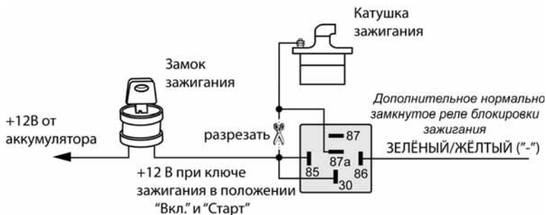
Схема подключения ЗЕЛЕНОГО/ЖЕЛТОГО провода для блокировки цепи зажигания автомобиля:
