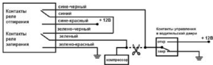
Схема подключения к пневматической системе запираания
