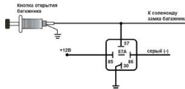
Схема подключения к соленоиду замка с отрицательной полярностью
