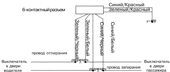
Схема 3. 5 (4) проводная система с переменной полярностью (большинство автомобилей Ford и Chrysler)
