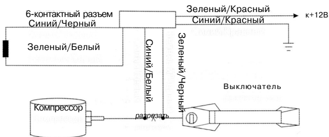
Схема 4. Вакуумная система центрального замка (Mercedes-Benz и Audi)
