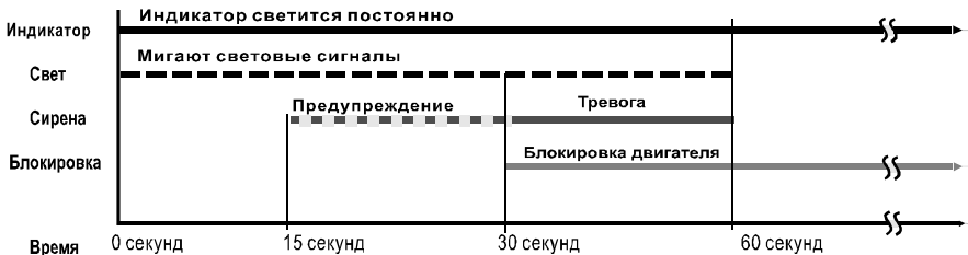
Временная диаграмма 1
